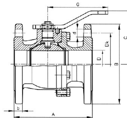
DN 65 - 200
