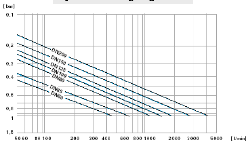
Nyomásvesztés diagram
